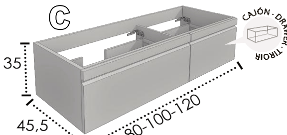
SIANI 35 1 CAJÓN / DRAWER / TIROIR
