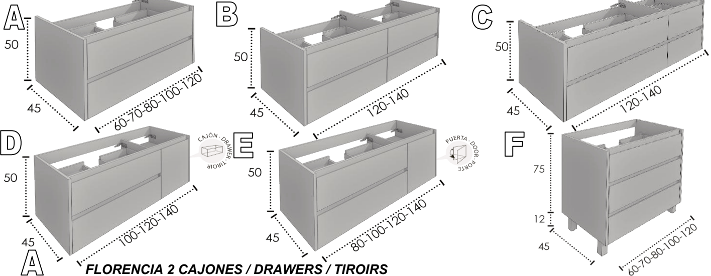
FLORENCIA 2 CAJONES / DRAWERS / TIROIRS
